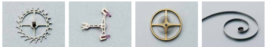
がんぎ車
